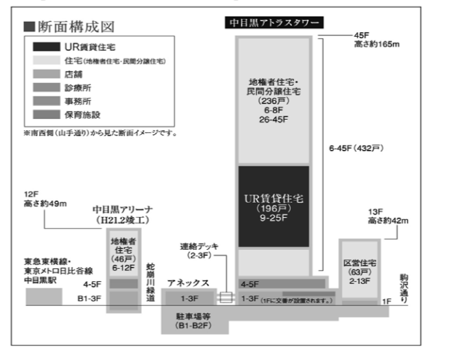
▼【ナカメアルカス断面構成図】独立行政法人都市再生機構発行「中目黒散歩」より
